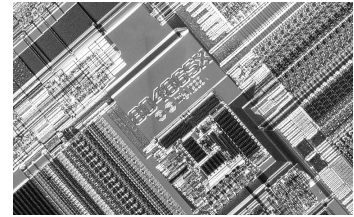
Figura 6. Interior del procesador 80486 de Intel.
