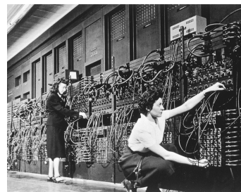
Figura 2 El ENIAC, Electronic Numerical Integrator and Computer (computador e integrador numérico electrónico), pesaba aproximadamente 30 toneladas, ocupaba 150 m 2 y consumía una potencia de 150 kW.
